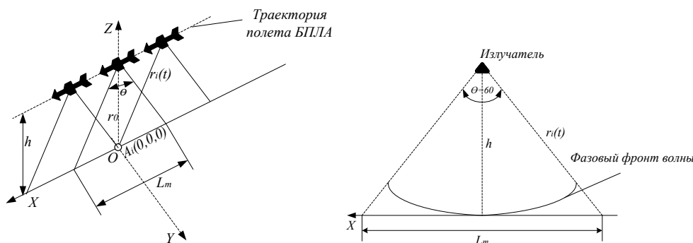
Рис. 2. Геометрия модели
