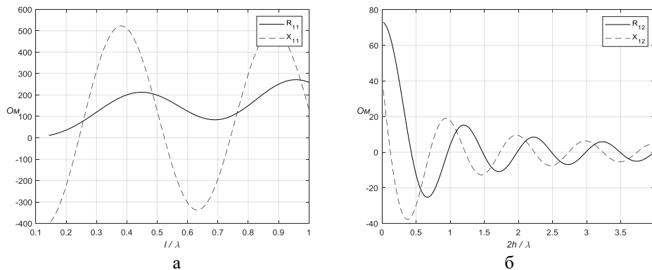
Рис. 2. Результаты верификации модели: значения величин Z_{11} (а) и Z_{12} (б) для частного случая: \alpha = 0 , \frac{l}{d} = 3000 и нулевого осевого сдвига диполей
