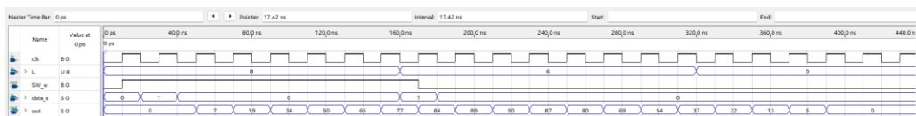
Рис. 2. Результат моделирования структуры управляемого РКИХ-фильтра с ИХ в виде окна Ханна в программе Quartus Prime
