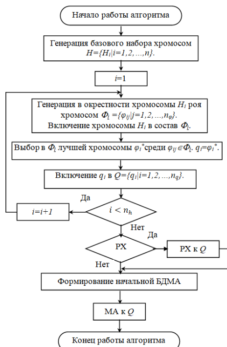
Рис. 1. Структура многоагентной системы построения паросочетания
