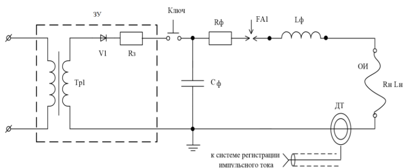
Рис. 7. Упрощенная принципиальная схема испытательной установки: ЗУ – зарядное устройство; Tr1 – трансформатор; V1 – вентиль высоковольтный; Rз – защитный резистор; Ключ – коммутатор подключения зарядного устройства к схеме; Cф – блок формирующий импульсных конденсаторов емкостного накопителя энергии; Rф – формирующий резистор; FA1 – управляемый коммутатор; Lф – формирующая индуктивность; ДТ – измерительный датчик тока; ОИ – объект испытаний
